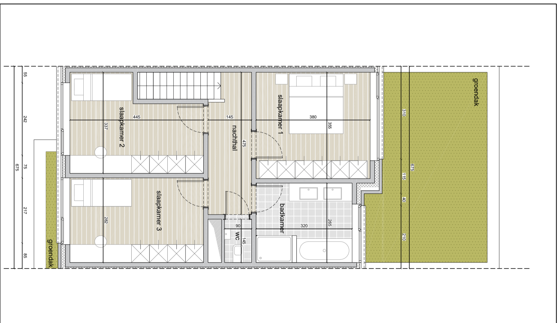
WONING 2 - VERDIEPING 1 schaal 1:75
